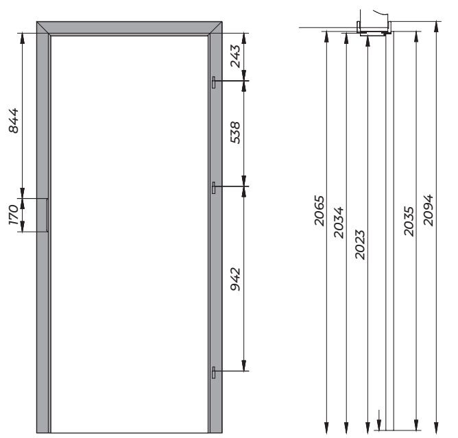
Ościeżnica panelowa OR
