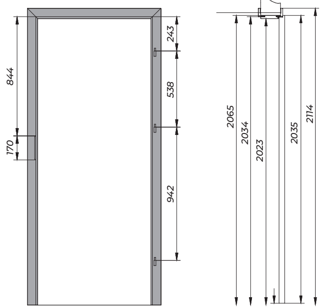
Ościeżnica panelowa OW
