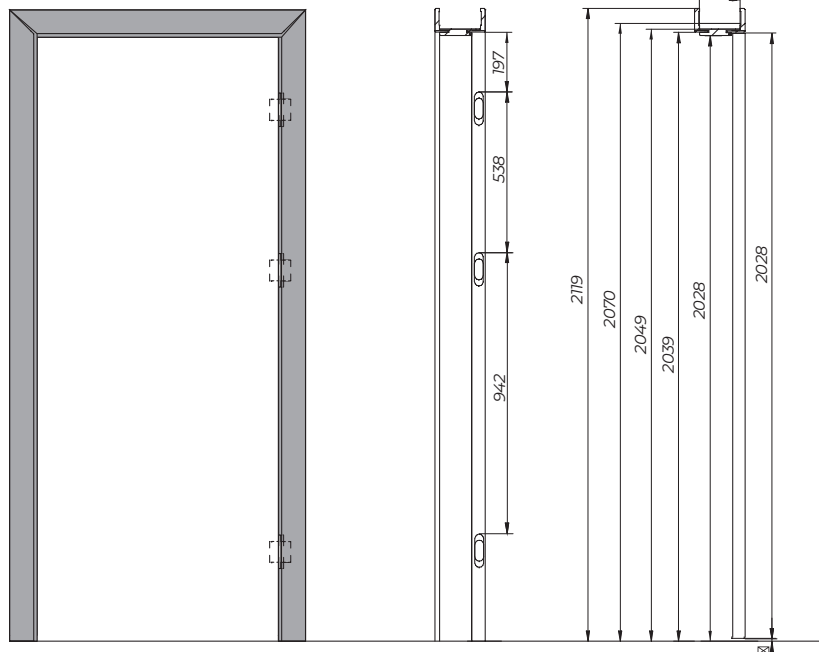
Ościeżnica panelowa OPB
