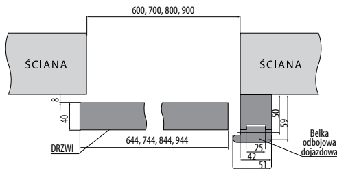
Rysunek systemu przesuwne go naścienne go bez zabudowy
