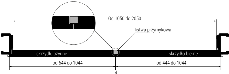
Przykładowe zewnętrzne wymiary ościeznicy w zależności od zastosowanej kombinacji skrzydeł drzwi
