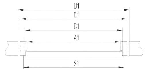
Wymiary ościeznic stałych (OS)
