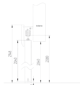
System przesuwny naścienny bez zabudowy
