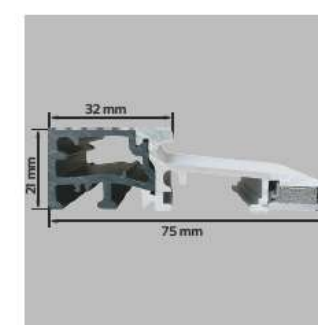
PRÓG ENERGO Z WKŁADKĄ TERMICZNĄ
