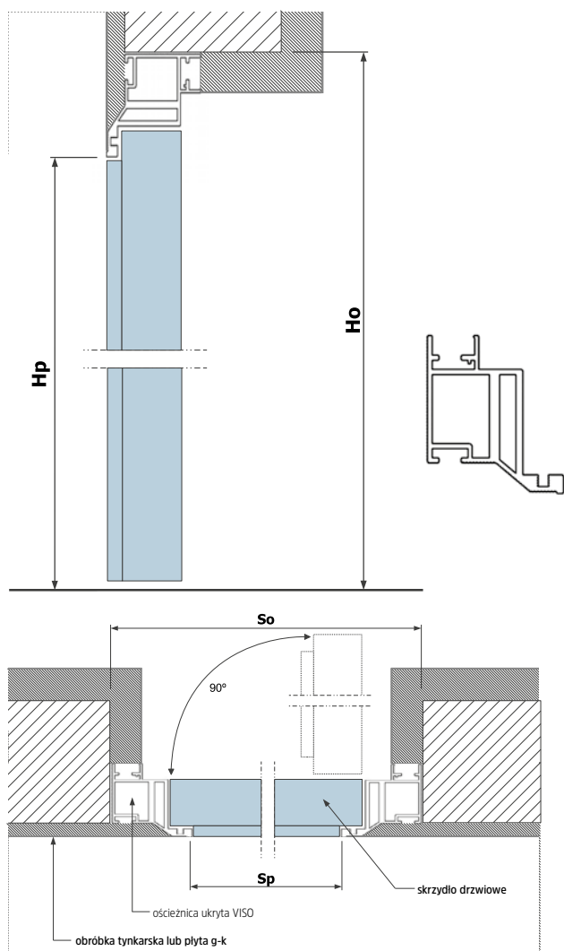
VISIO 40 - WEWNĘTRZNE
