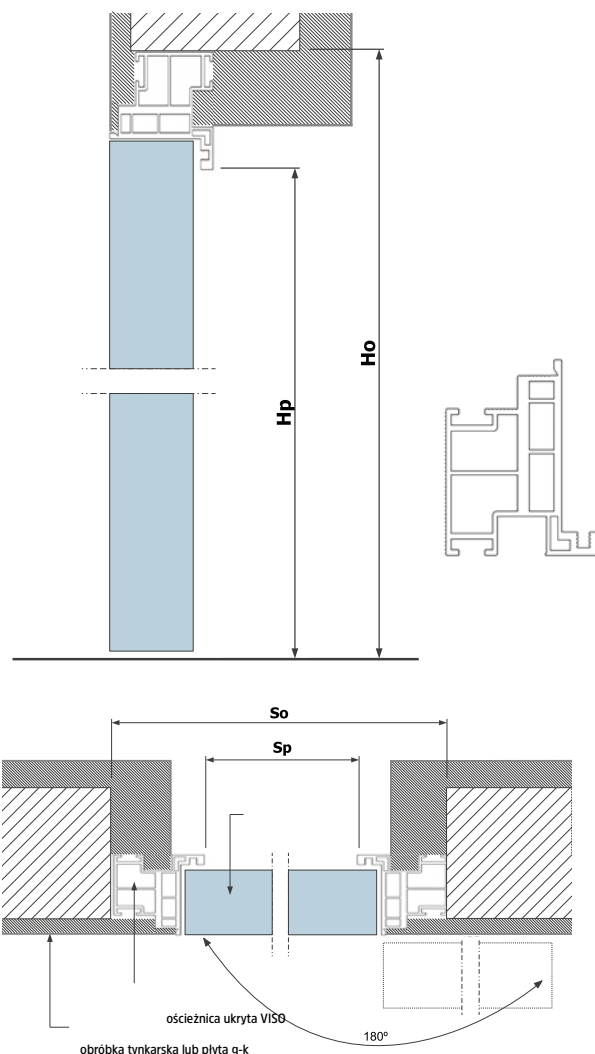
VISIO 40 - ZEWNĘTRZNE
