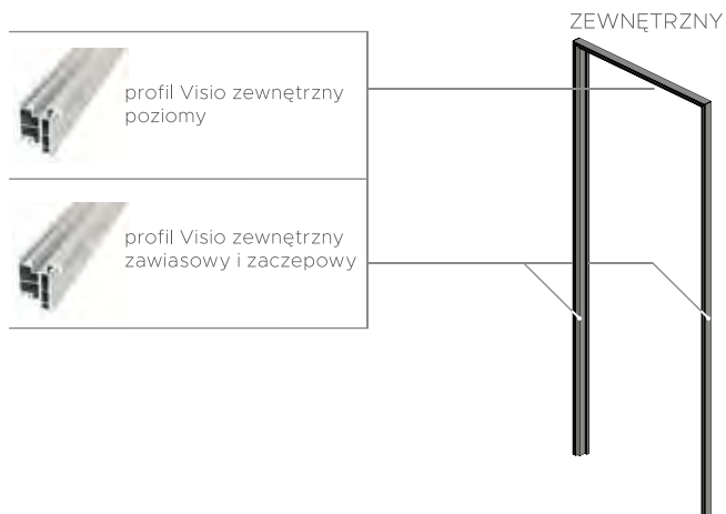
ELEMENTY OPCJONALNE
