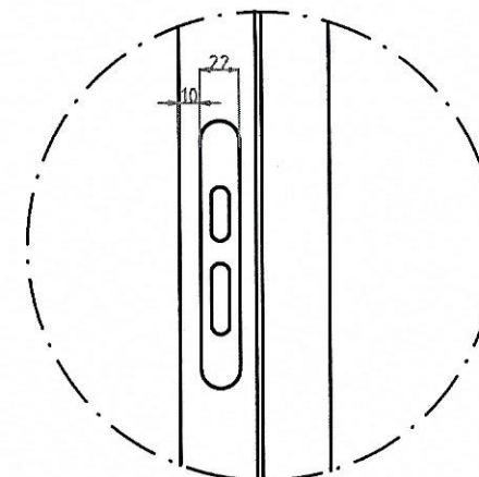
SZCZEGÓŁ B
