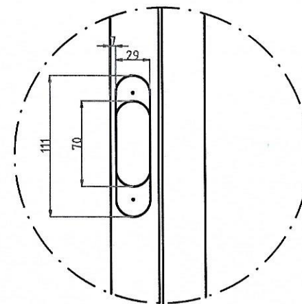
SZCZEGÓŁ A
