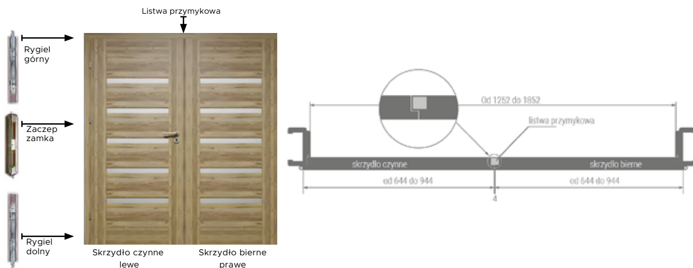
Skrzydła drzwi podwójne z listwą przyrywkową
