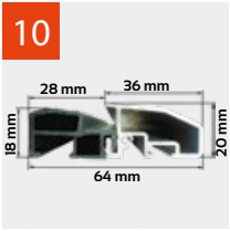
CIEPŁY PRÓG ALUMINIOWY Z WKŁADKĄ PVC
