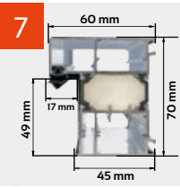
CIEPŁA OŚCIEŻNICA Z IZOLACJĄ
