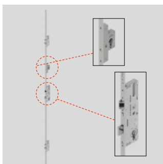
[ ZAMEK LISTWOWY Z DODATKOWYM GÓRNYM ZAMKIEM Z REGULOWANYMI ZACZEPAMI W OŚCIEŻNICY TO ROZWIĄZANIE POSIADA ZAMEK CZTEROPUNKTO- WY-RYGŁOWY W KOMPLECIE Z WKŁADKĄ ORAZ GÓRNĄ WKŁADKO-GAŁKĄ, KLAMKĄ, ROZETĄ GÓRNĄ
