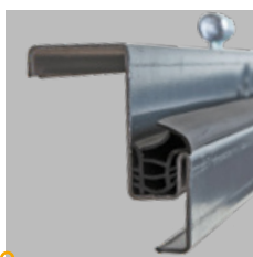
PRZEKRÓJ OŚCIEŻNICY KĄTOWEJ Z USZCZELKĄ
