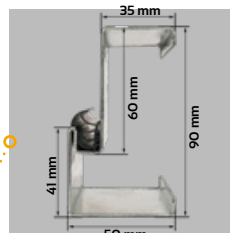
PRZĘKRÓJ OŚCIEŻNICY SYMETRYCZNEJ Z USZCZELKĄ
